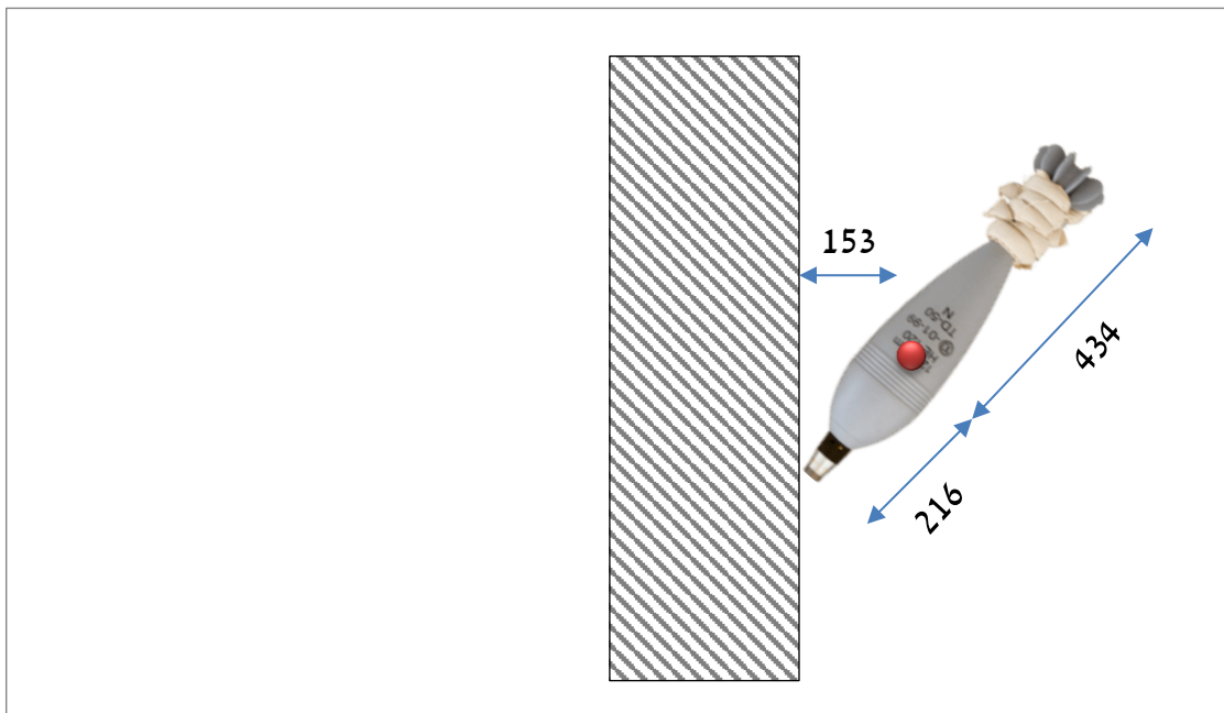
איור 7 - פגז 120 מ"מ – זווית פגיעה
